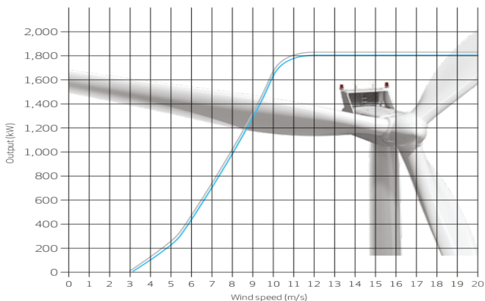
Rycina 1. Krzywa mocy turbiny VESTAS V100 – 1.8 MW (Źródło: www.vestas.com )
